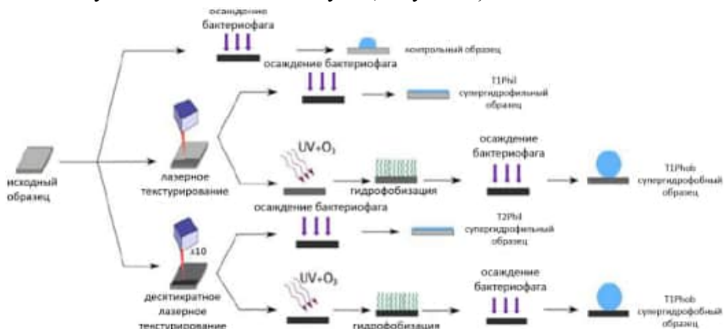
Рисунок 1 - Схема изготовления исследуемых образцов из алюминия, меди, нержавеющей стали, магния
